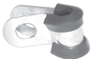
JC REI: 23178 | OR: 813.936 Descrição: Braçadeira Ø 13,0mm Aplicação: P-93 F-113 K-113 R-113 T-113 R-143 C-113/114/124/94/94I/94H/94U 124E 124I
