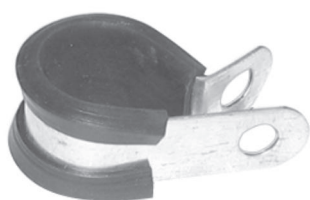
JC REI: 23170 | OR: 804.583 Descrição: Braçadeira Ø 32,0mm Aplicação: P-93 F-113 K-113 R-113 R143 C-113/94/94 U/124/124 E/124 I/114/94 I
