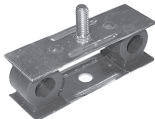
JC REI: 23147 | OR: 366.006 Descrição: Coxim da Lanterna Tomada de Reboque Aplicação: T-112 / 113 R-142 / 143 P-93
