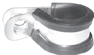
JC REI: 23179 | OR: 813.937 Descrição: Abraçadeira Ø 16,0mm Aplicação: P-93 F-113 K-113 R-113 T-113 R-143 C-113 / 114 / 124 / 94 / 94 I 94-H 94-U 124 E / 124 I
