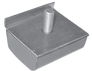
JC REI: 23145 | OR: 361.243 Descrição: Coxim Batente Suspensão a Ar da Cabine Aplicação: T-113 T-143
